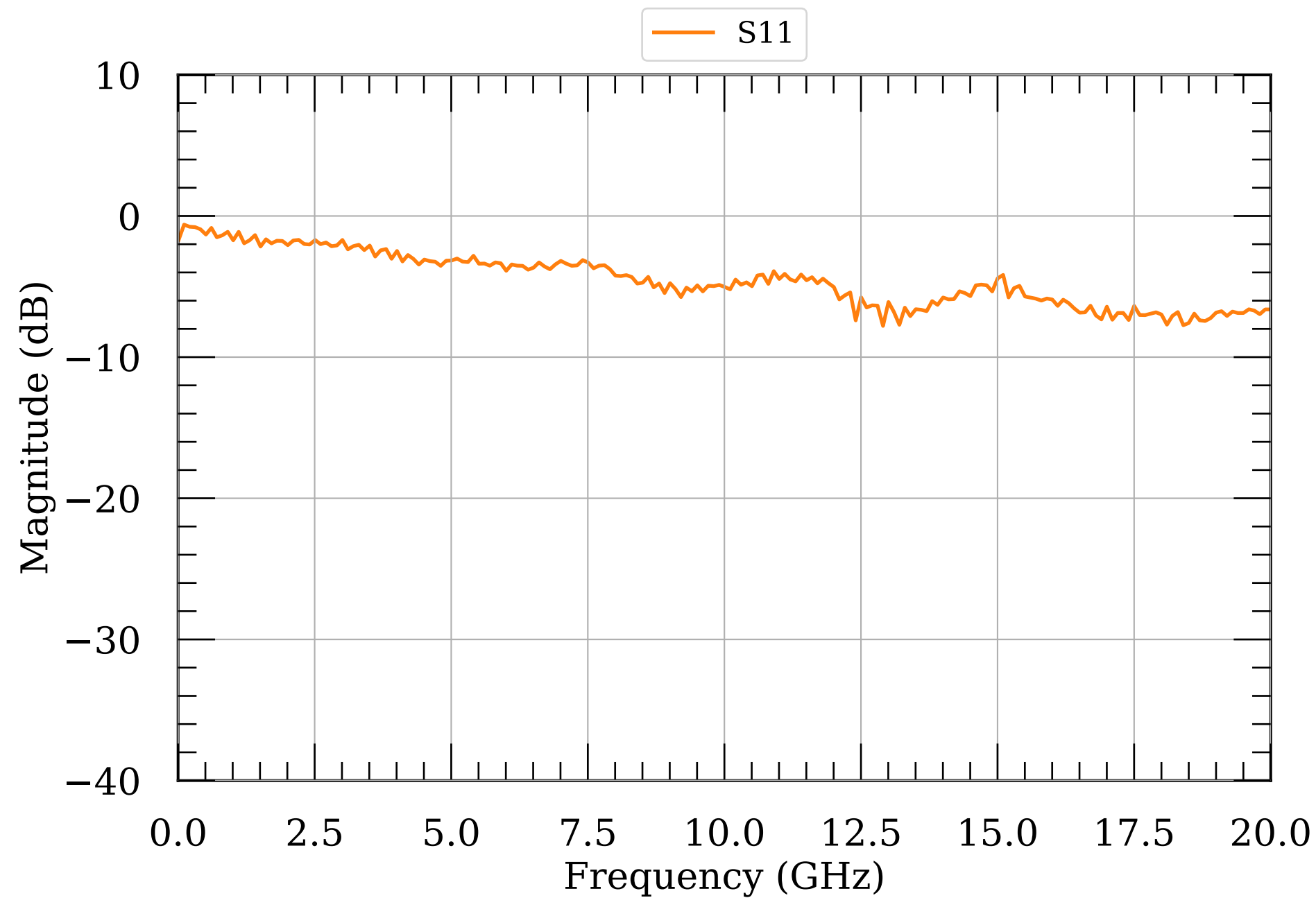
LNA S-params module063
